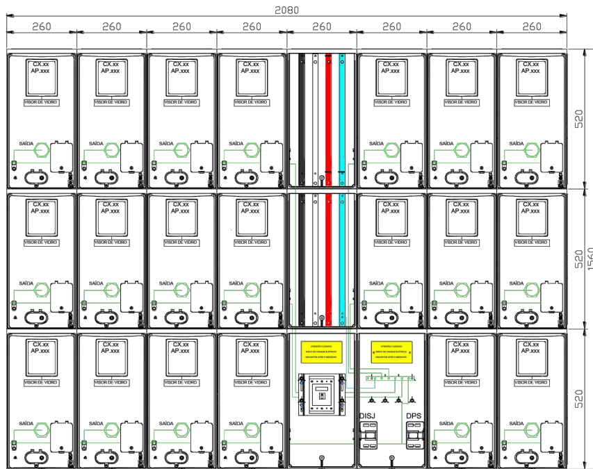
Montagem para instalação de 13 até 20 medidores Disjuntor geral até 200A
