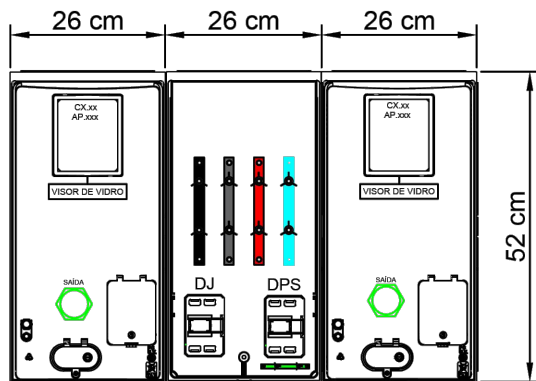
Montagem para instalação de até 02 medidores disjuntor geral até 70A (Obrigatório execução em mureta)
