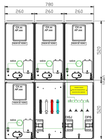
Montagem para instalação de até 04 medidores disjuntor geral até 70A
