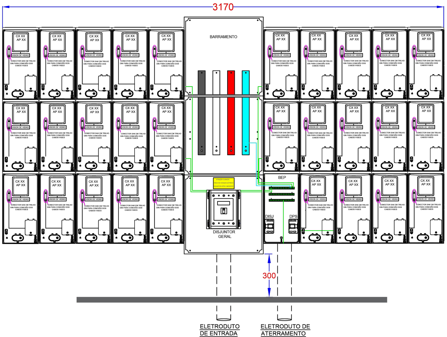
Montagem para instalação de 21 até 33 medidores
